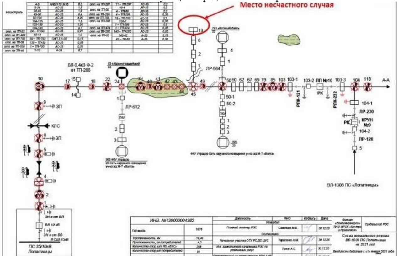
Место несчастного случая на схеме нормального режима ЛЭП.
