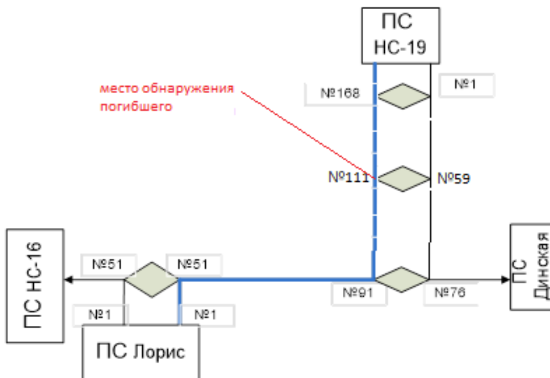
Место несчастного случая на схеме ЛЭП.
