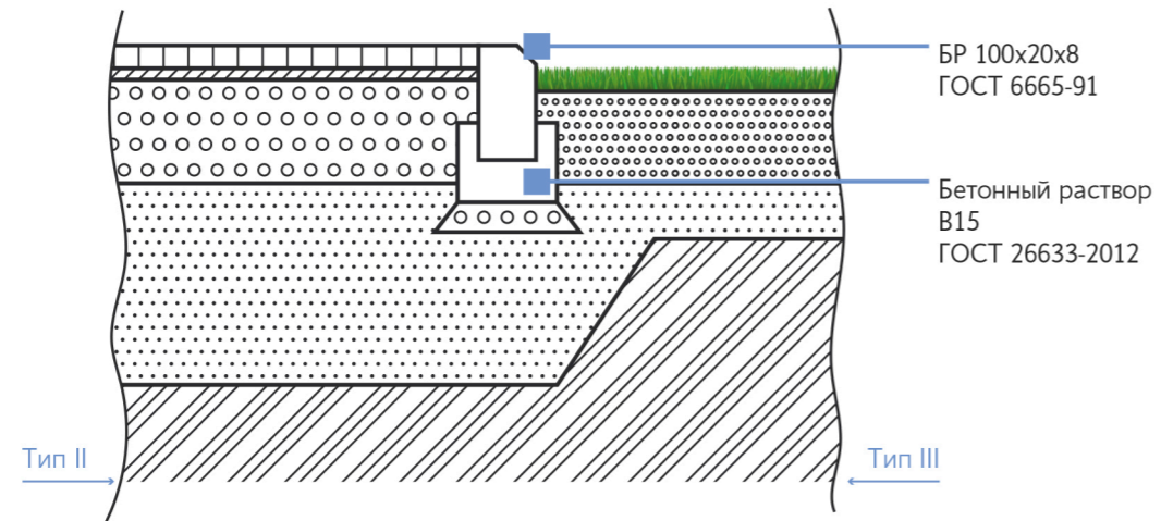
УЗЕЛ СОПРЯЖЕНИЯ 1
