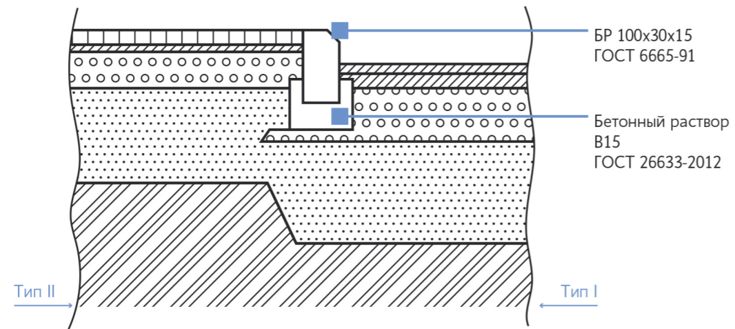
УЗЕЛ СОПРЯЖЕНИЯ 2
